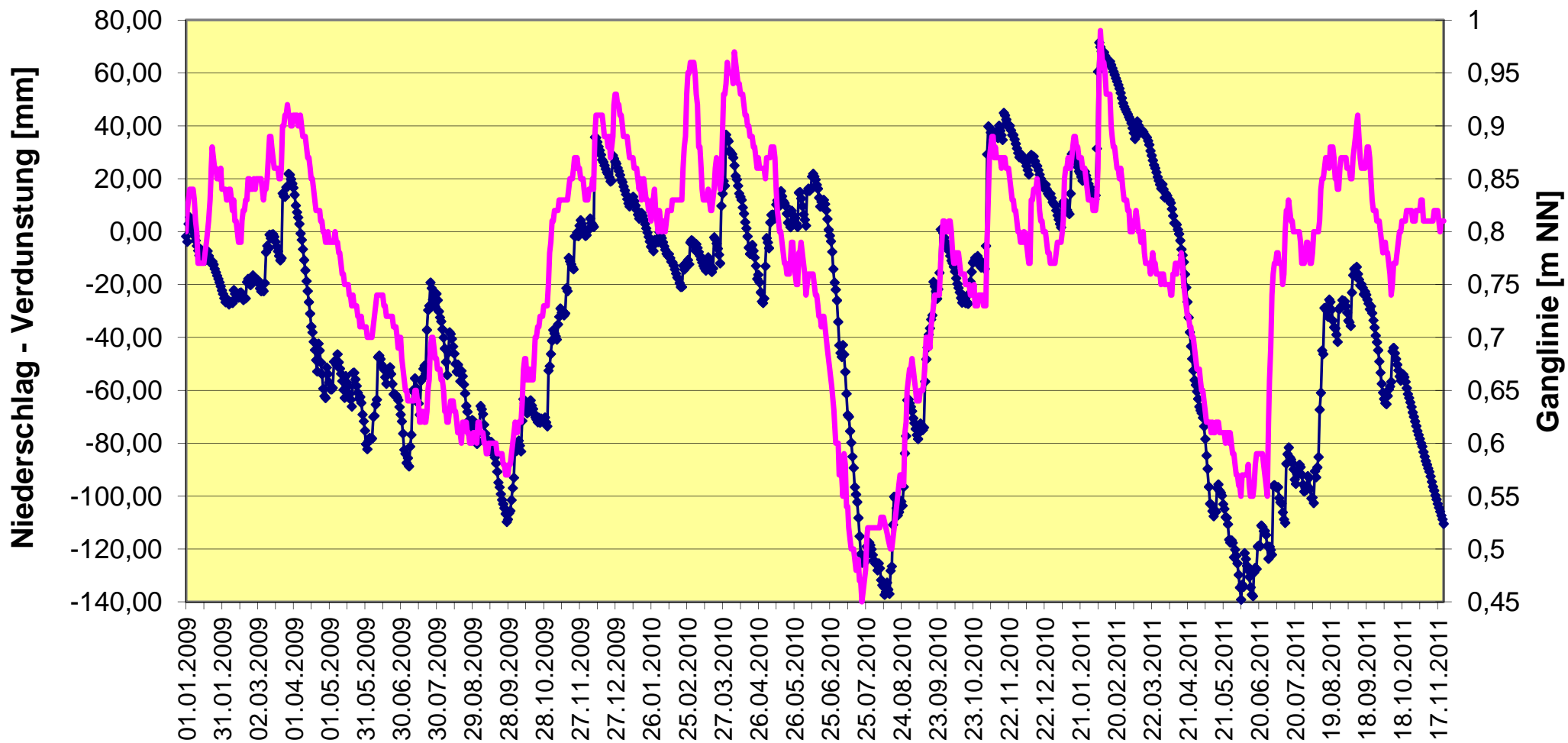
Vergleich Niederschläge minus Verdunstung (aufsummierte Abweichungen vom Tagesmittelwert des Zeitraums, blaugepunktet) und Ganglinie der Messstelle 8469 in HH-Neuwiedenthal, ab 01.01.2009, Stand 22.11.11
