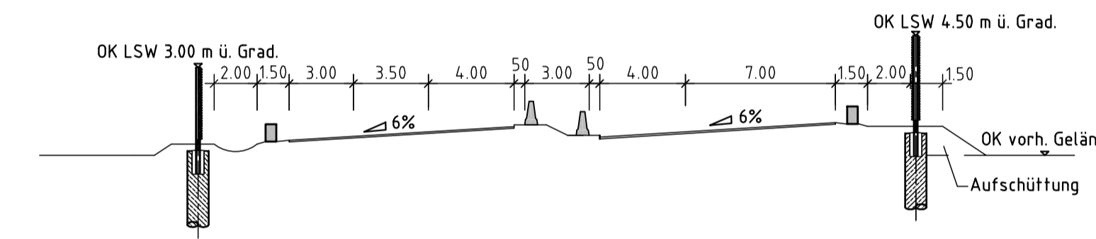
Querschnitt M. 1:250
