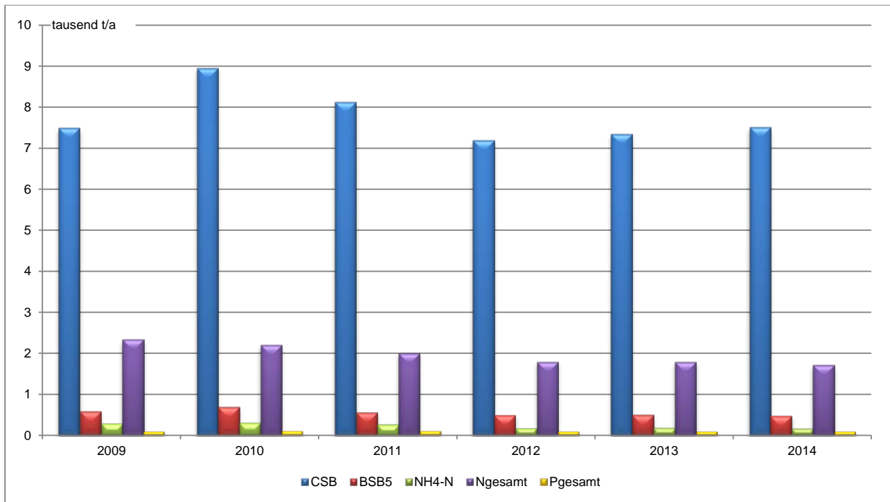
Abbildung 2: Abwasserschmutzfrachten
