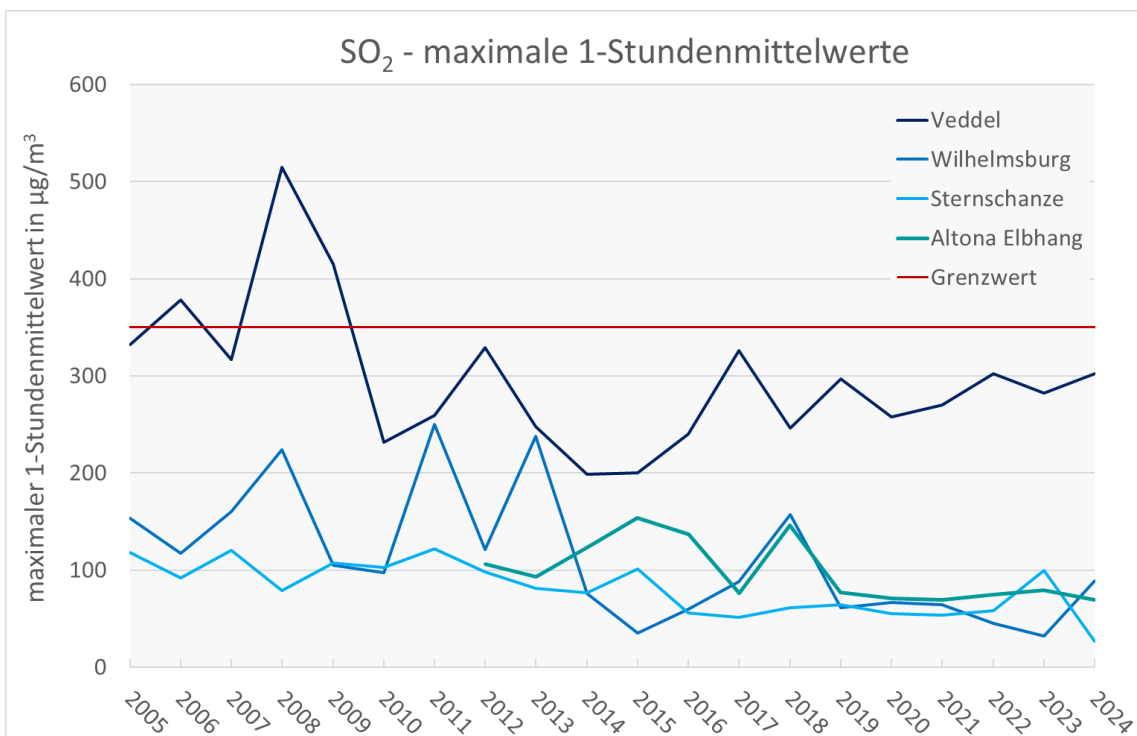
Abbildung 23: maximale 1-Stundenmittelwerte der Schwefeldioxidkonzentrationen in \mu\text{g}/\text{m}^3 der Jahre 2005 bis 2024 an Messstationen zum Vollzug der 39. BImSchV in Hamburg.
