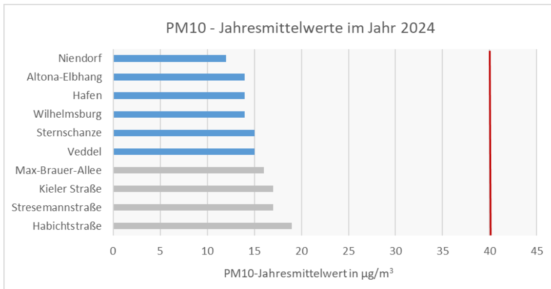
Abbildung 10: Jahresmittelwerte der PM10-Konzentration in \mu\text{g}/\text{m}^3 an den Messstationen zum Vollzug der 39. BImSchV in Hamburg im Jahr 2024.
