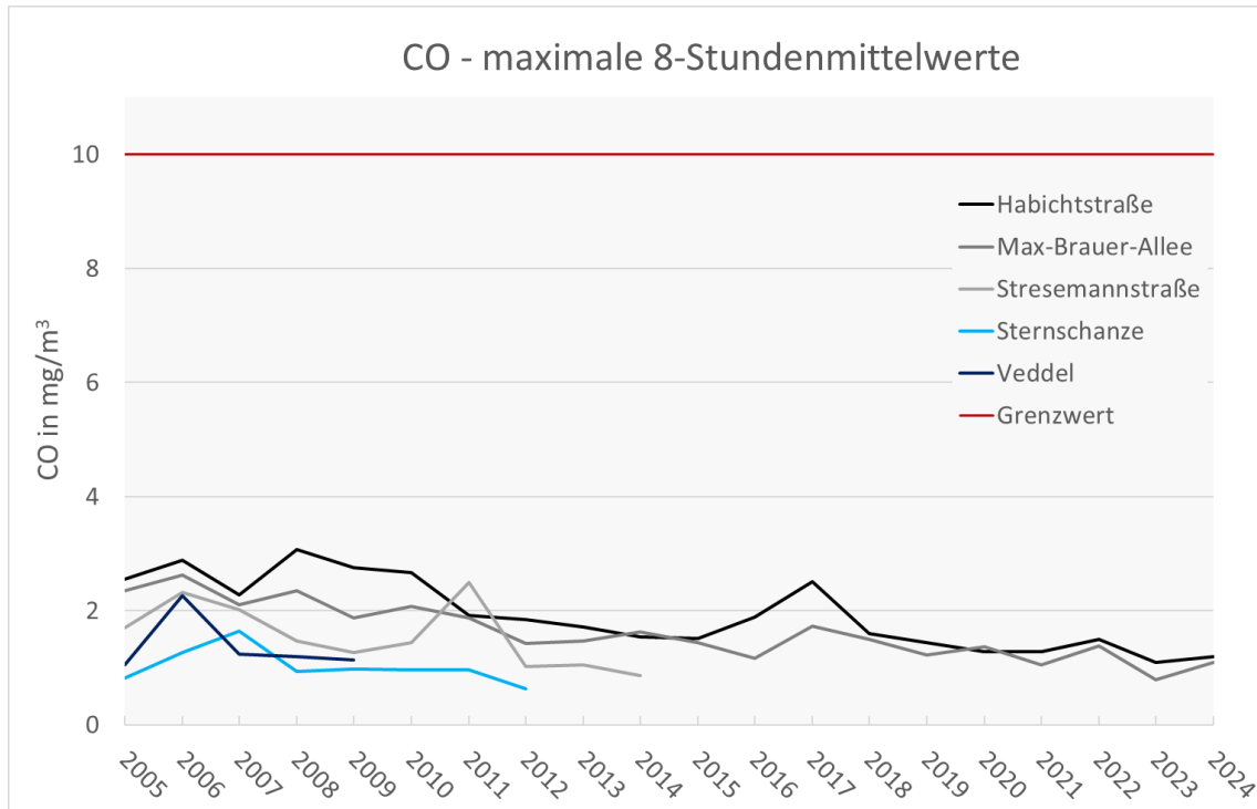
Abbildung 26: Maximale 8-Stundenmittelwerte der Kohlenstoffmonoxid-Konzentrationen in mg/m 3 der Jahre 2005 bis 2024 an Messstationen zum Vollzug der 39. BImSchV in Hamburg.
