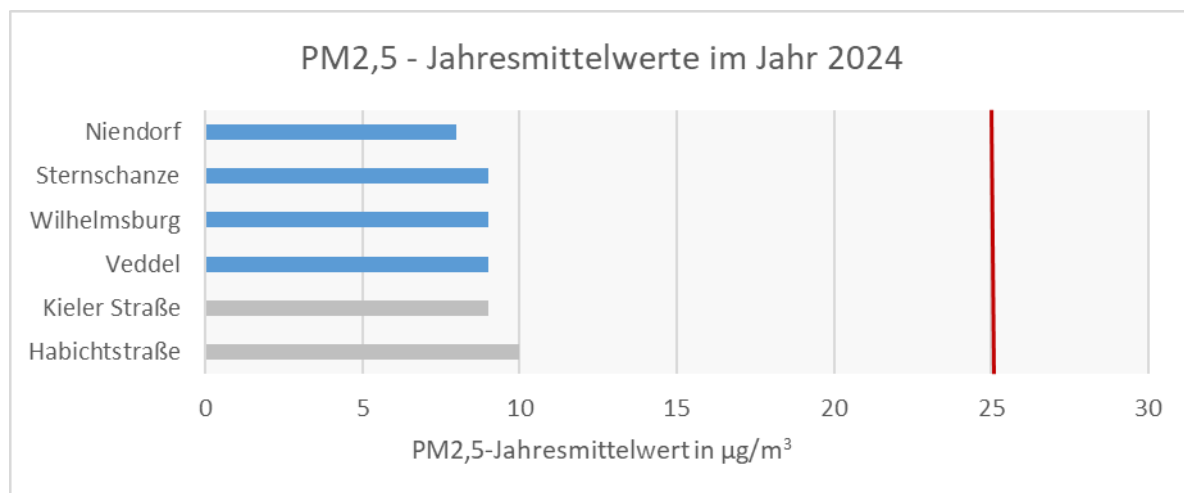
Abbildung 14: Jahresmittelwerte der PM2,5-Konzentration in \mu\text{g}/\text{m}^3 an den Messstationen zum Vollzug der 39. BImSchV in Hamburg im Jahr 2024.
