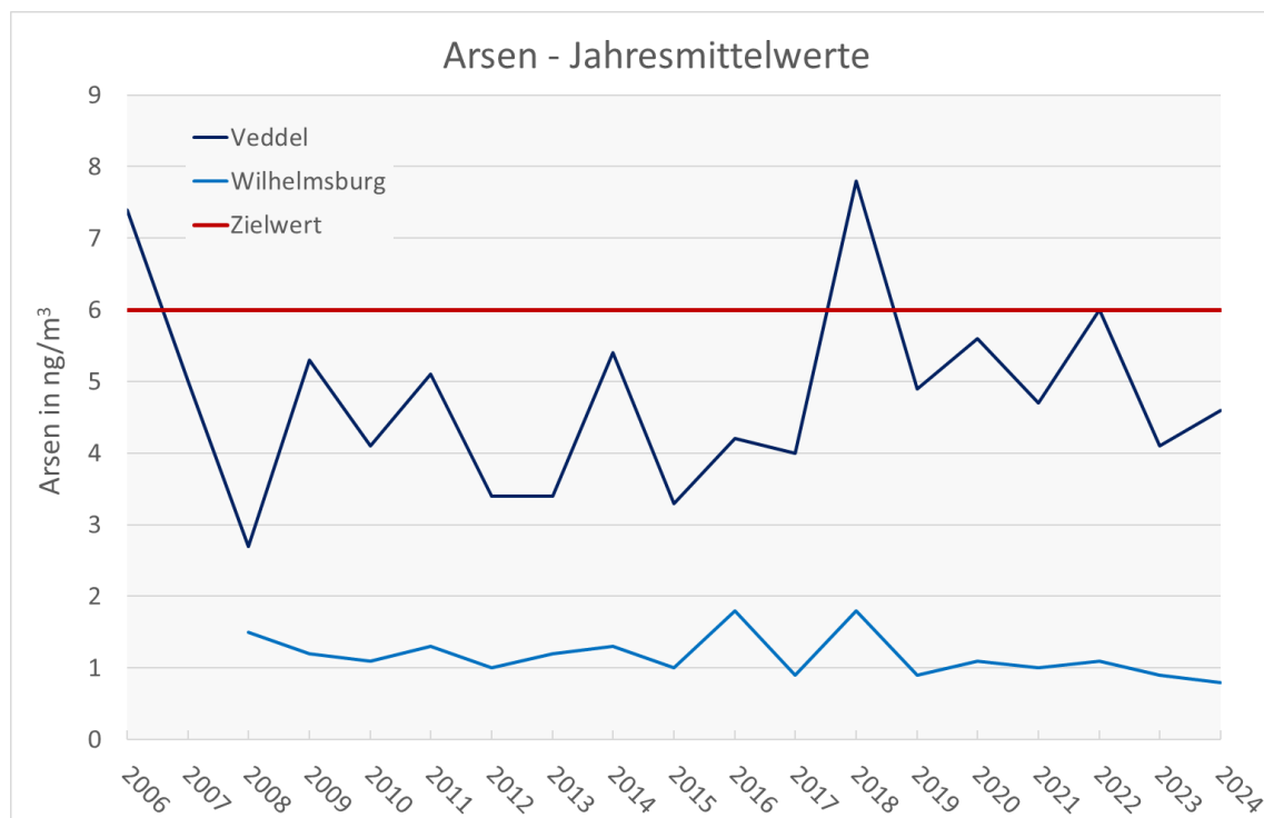
Abbildung 30: Jahresmittelwerte der Konzentration an Arsen in PM10 in \text{ng/m}^3 der Jahre 2006 bis 2024 an Messstationen zum Vollzug der 39. BImSchV in Hamburg.
