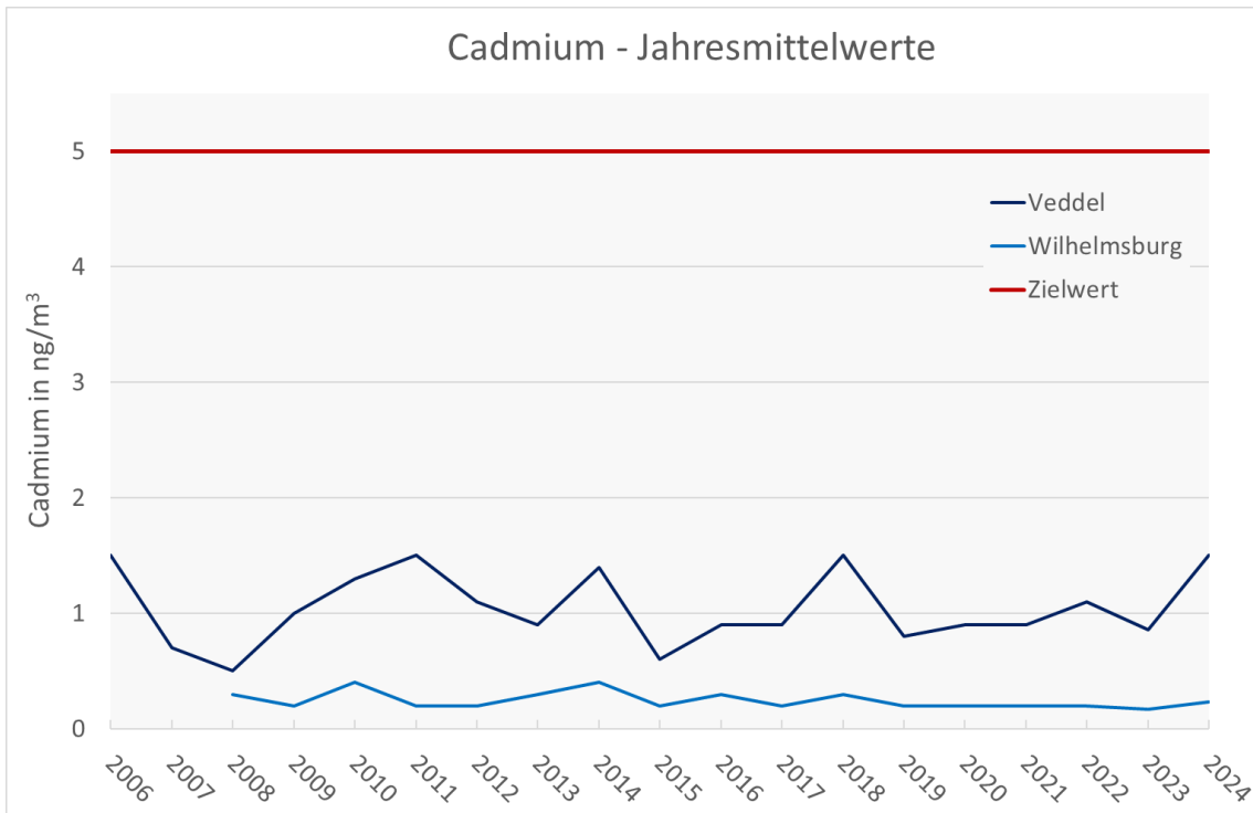
Abbildung 31: Jahresmittelwerte der Konzentration an Cadmium in PM10 in ng/m 3 der Jahre 2006 bis 2024 an Messstationen zum Vollzug der 39. BImSchV in Hamburg.
