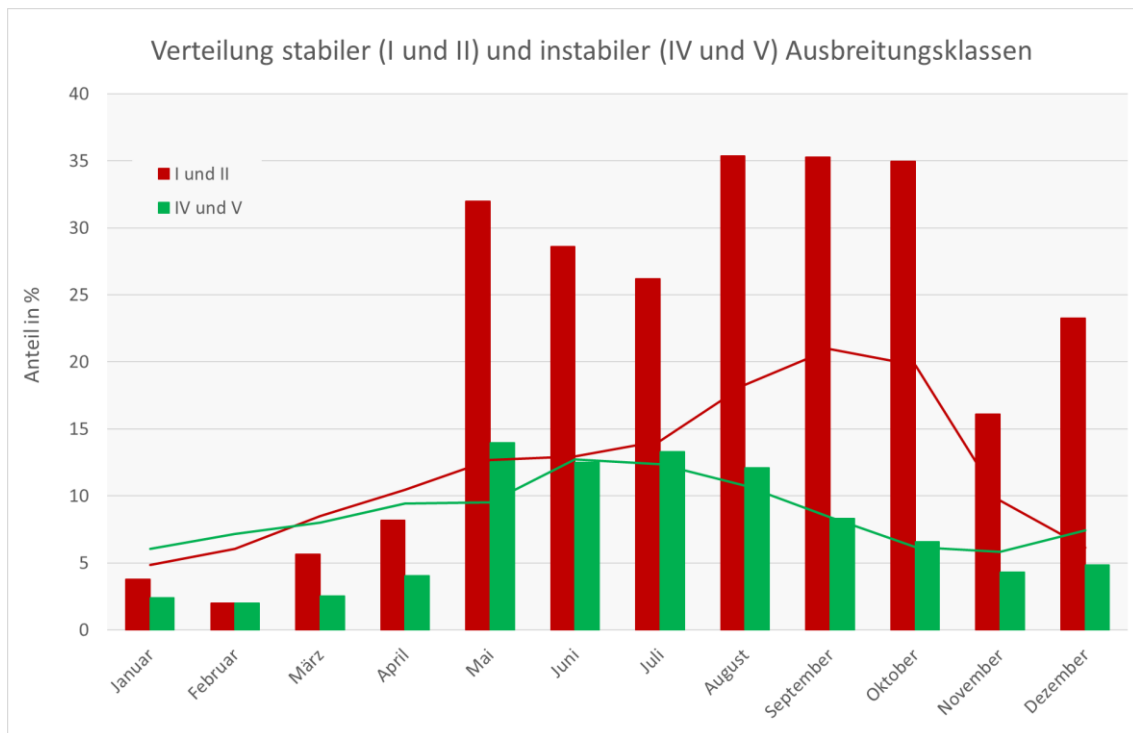
Abbildung 5: Verteilung stabiler und instabiler Ausbreitungsklassen in % im Jahr 2024 (Balken) und Mittelwerte der Jahre 2006-2024 (Linien) am Wettermast Hamburg. Datenquelle: Universität Hamburg.
