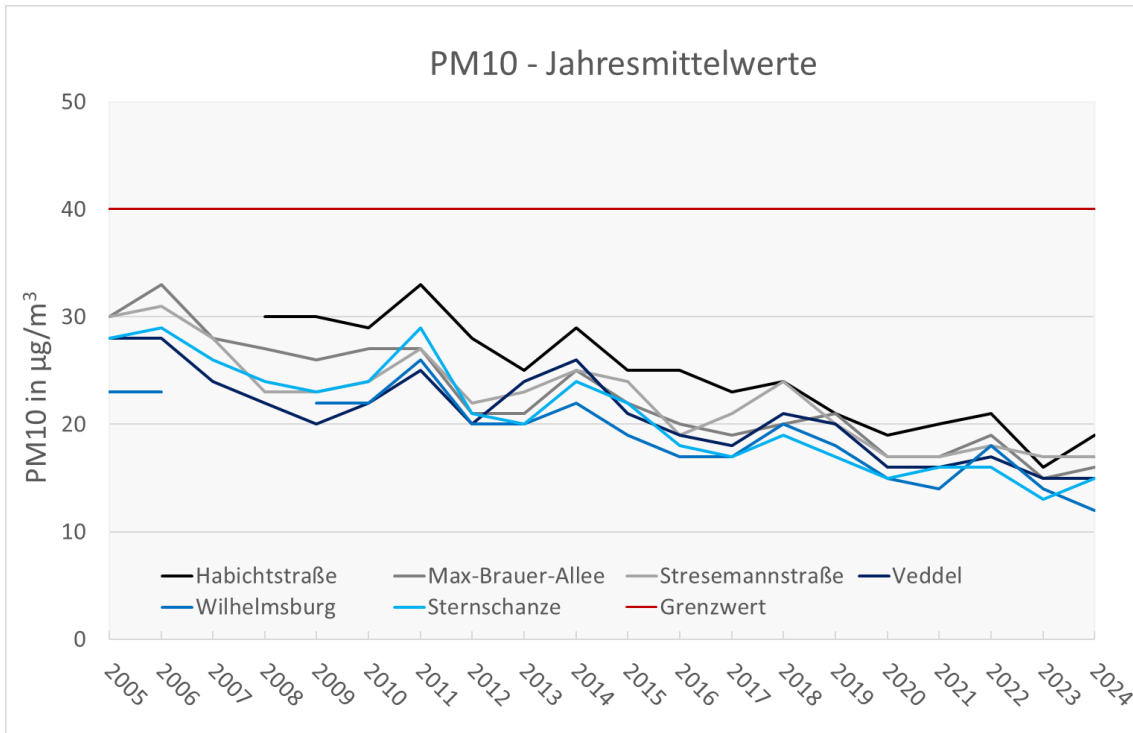
Abbildung 12: Jahresmittelwerte der PM10-Konzentration in \mu\text{g}/\text{m}^3 der Jahre 2005 bis 2024 an Messstationen zum Vollzug der 39. BImSchV in Hamburg.
