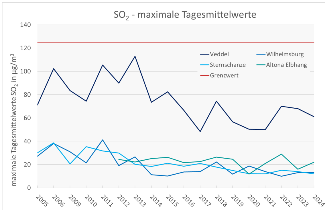
Abbildung 24: Maximale Tagesmittelwerte der Schwefeldioxidkonzentration in µg/m 3 der Jahre 2005 bis 2024 an Messstationen zum Vollzug der 39. BImSchV in Hamburg.
