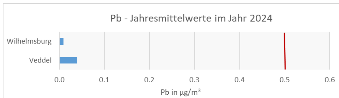
Abbildung 28: Jahresmittelwerte der Pb-Konzentration in PM10 in \mu\text{g}/\text{m}^3 an den Messstationen zum Vollzug der 39. BImSchV in Hamburg im Jahr 2024.
