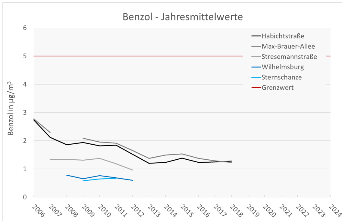
Abbildung 27: Jahresmittelwerte der Benzolkonzentration in \mu\text{g}/\text{m}^3 der Jahre 2006 bis 2018 an Messstationen zum Vollzug der 39. BImSchV in Hamburg.
