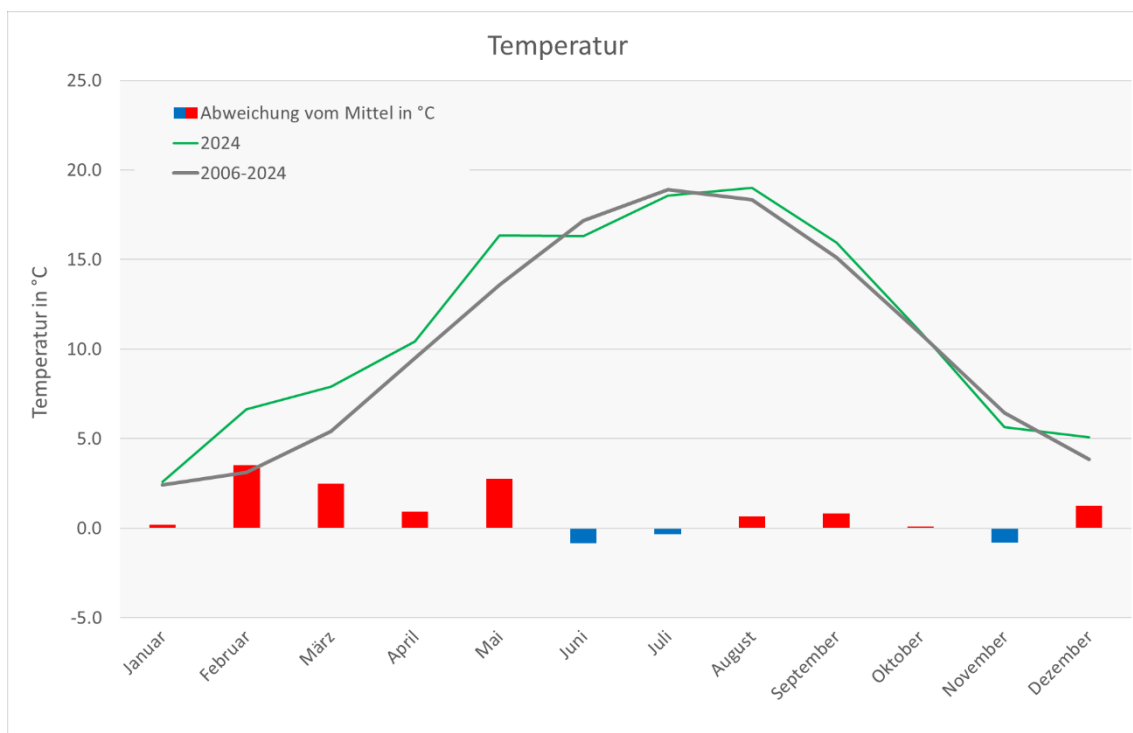
Abbildung 2: Monatsmittelwerte der Temperatur in °C am Wettermast Hamburg im Jahr 2024 (grüne Linie), Mittelwert der Jahre 2006-2024 (graue Linie) und den Abweichungen des Jahres 2024 vom Mittelwert der Jahre 2006-2024 (rote und blaue Balken). Datenquelle: Universität Hamburg.
