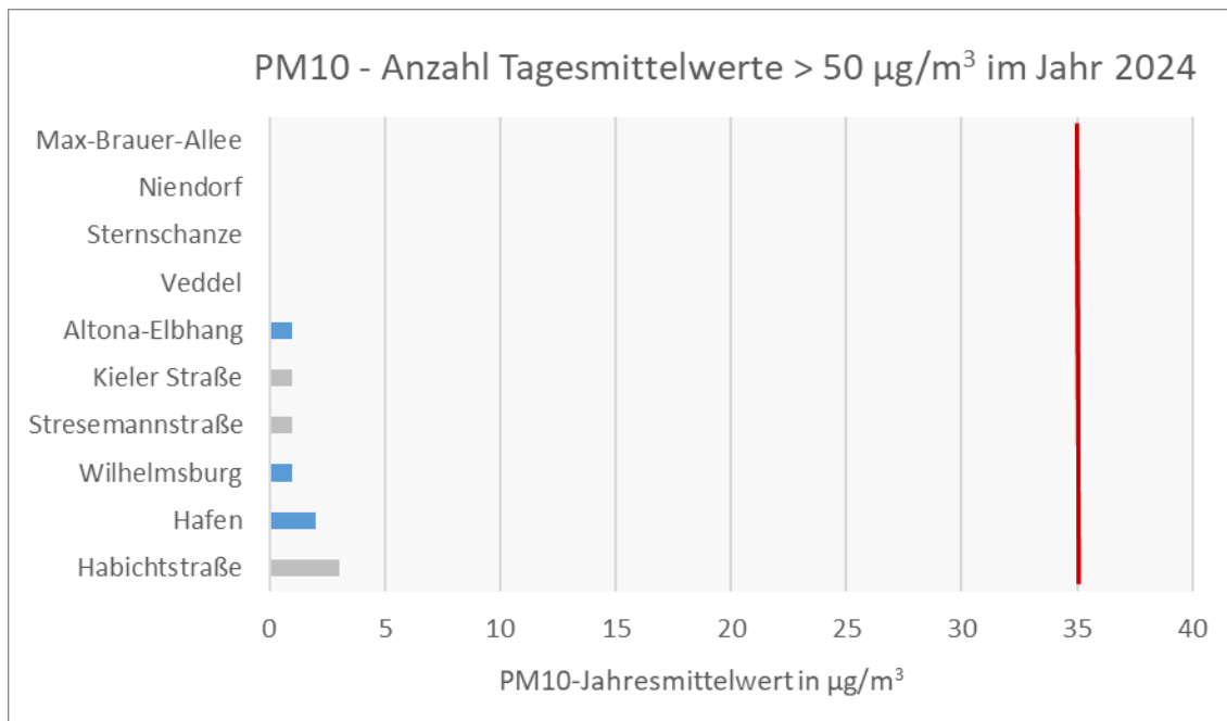
Abbildung 11: Anzahl an Tagesmittelwerte mit PM10-Konzentrationen > 50 \mu\text{g}/\text{m}^3 an den Messstationen zum Vollzug der 39. BImSchV in Hamburg im Jahr 2024.
