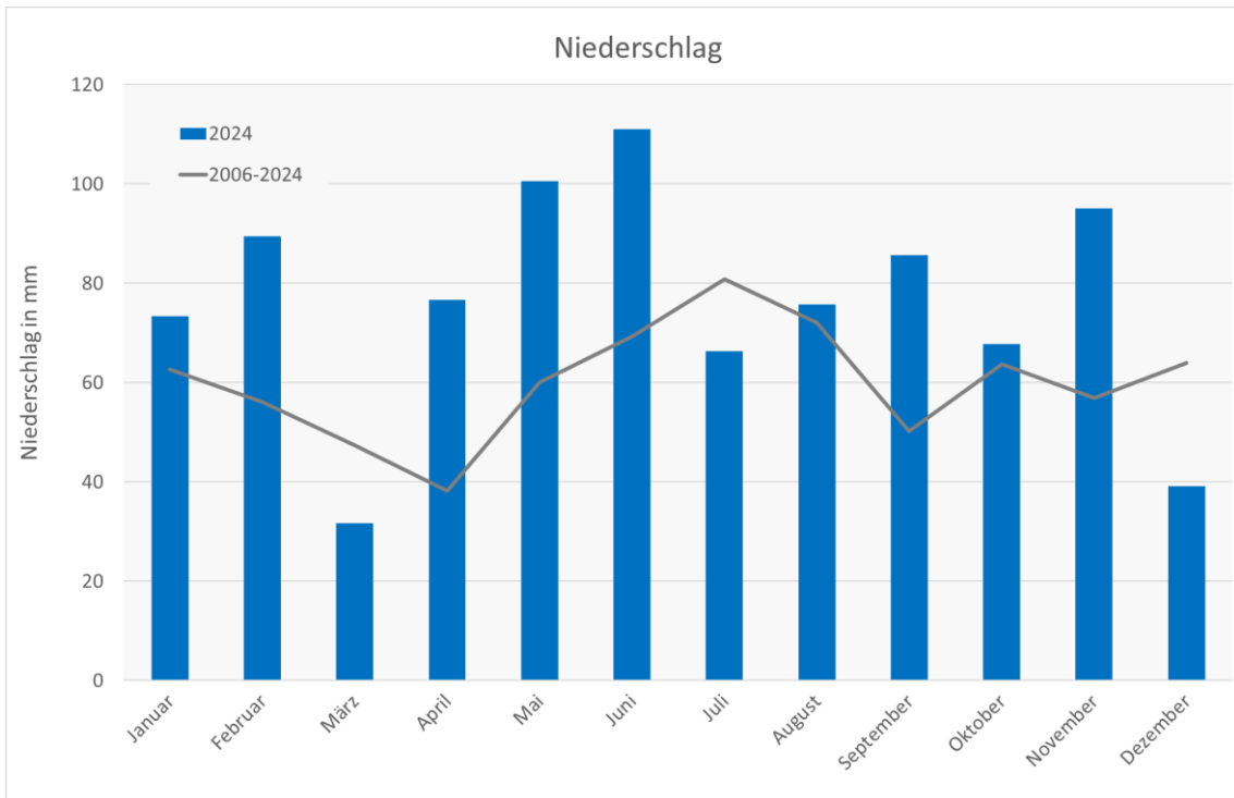
Abbildung 3: Monatssummen an Niederschlag in mm am Wettermast Hamburg im Jahr 2024 (blaue Balken) und Mittelwert der Jahre 2006-2024 (graue Linie). Datenquelle: Universität Hamburg.
