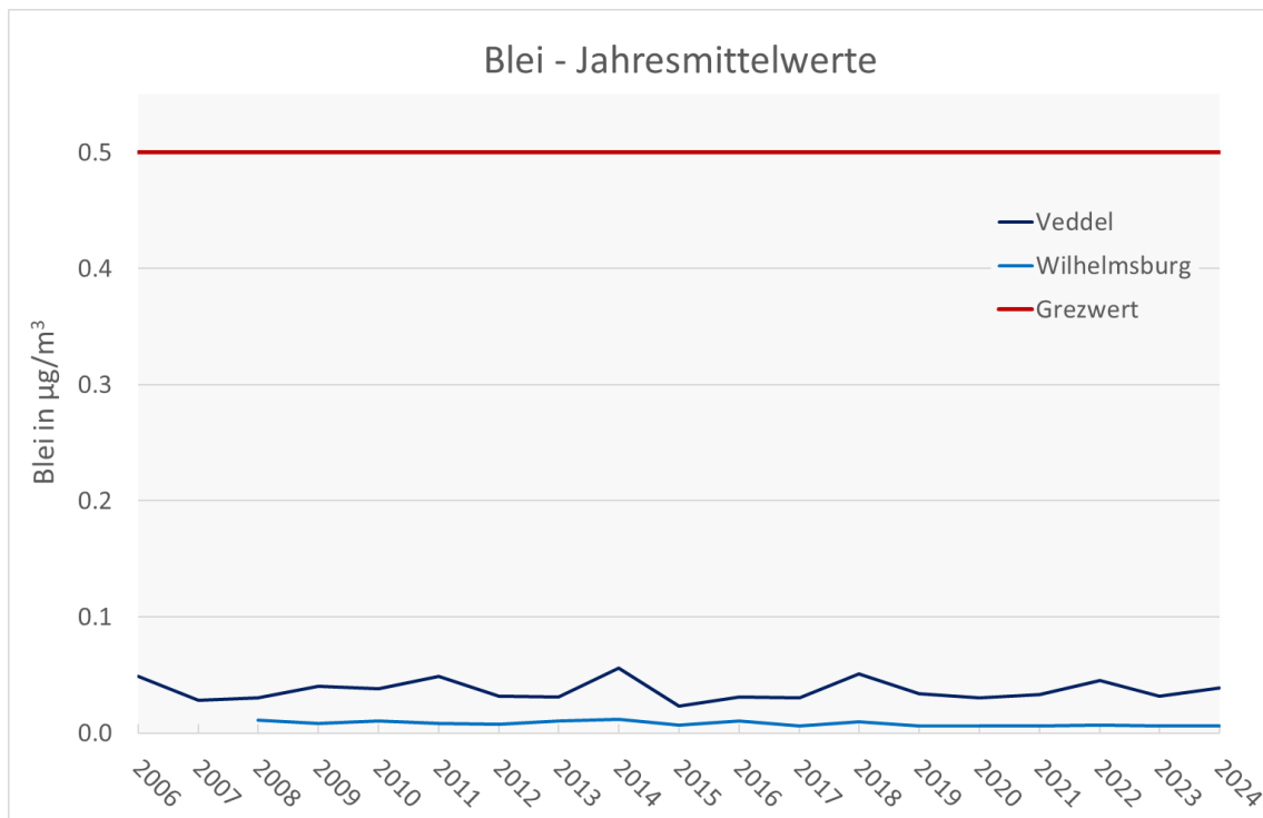
Abbildung 29: Jahresmittelwerte der Konzentration an Blei in PM10 in \mu\text{g}/\text{m}^3 der Jahre 2006 bis 2024 an Messstationen zum Vollzug der 39. BImSchV in Hamburg.
