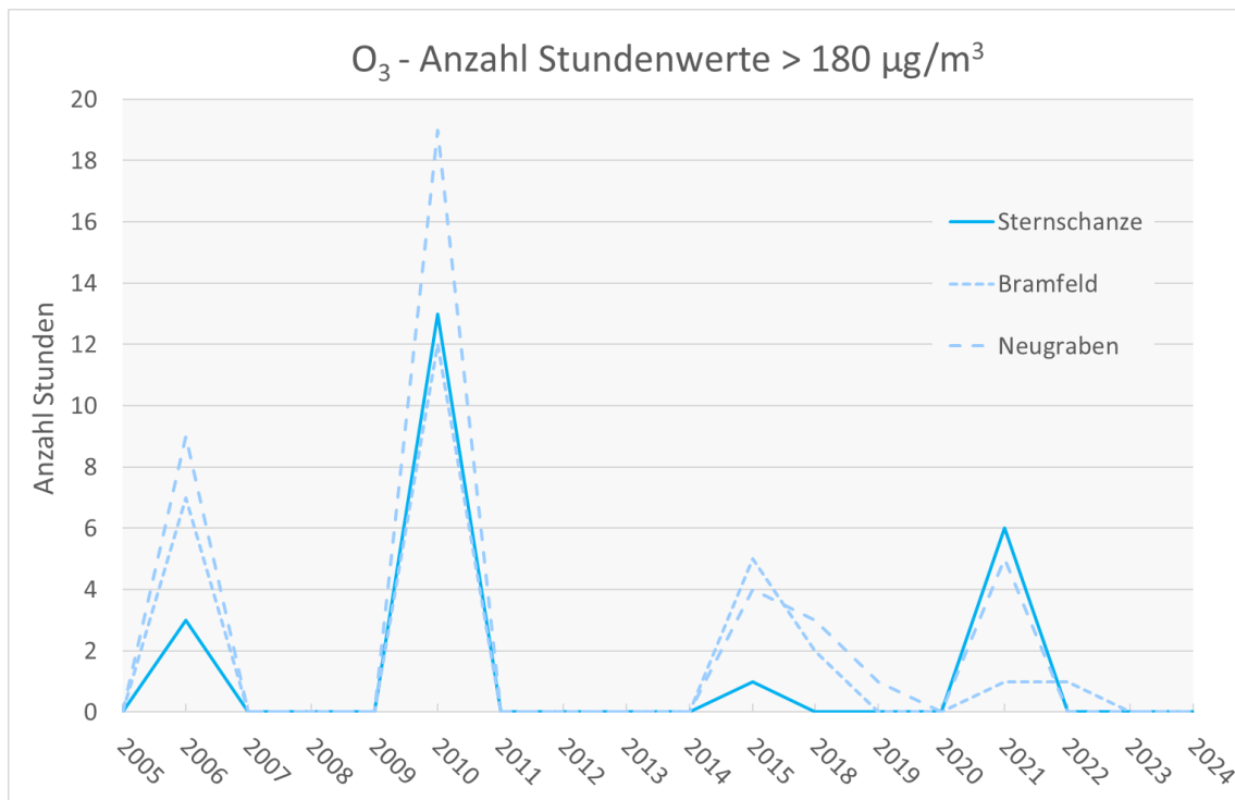
Abbildung 20: Anzahl an 1-Stundenmittelwerten mit bodennahen Ozonkonzentrationen > 180 µg/m³ (Informationsschwelle) der Jahre 2005 bis 2024 an Messstationen zum Vollzug der 39. BImSchV in Hamburg.
