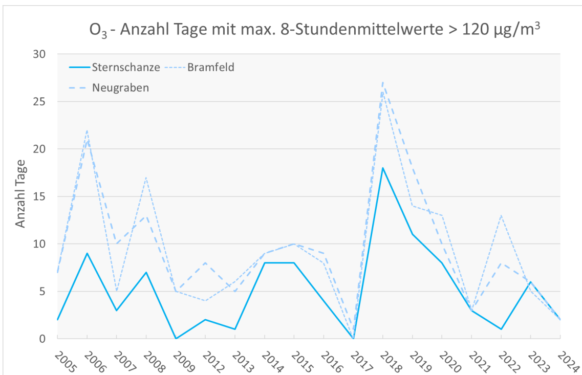
Abbildung 19: Anzahl an Tagen mit maximalen 8-Stundenmittelwerten mit bodennahen Ozonkonzentrationen > 120 \mu\text{g}/\text{m}^3 der Jahre 2005 bis 2024 an Messstationen zum Vollzug der 39. BImSchV in Hamburg.
