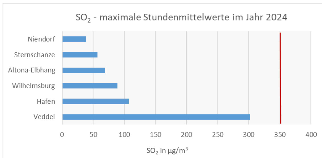
Abbildung 22: Maximale 1-Stundenmittelwerte der Schwefeldioxidkonzentrationen in \mu\text{g}/\text{m}^3 an den Messstationen zum Vollzug der 39. BImSchV in Hamburg im Jahr 2024.
