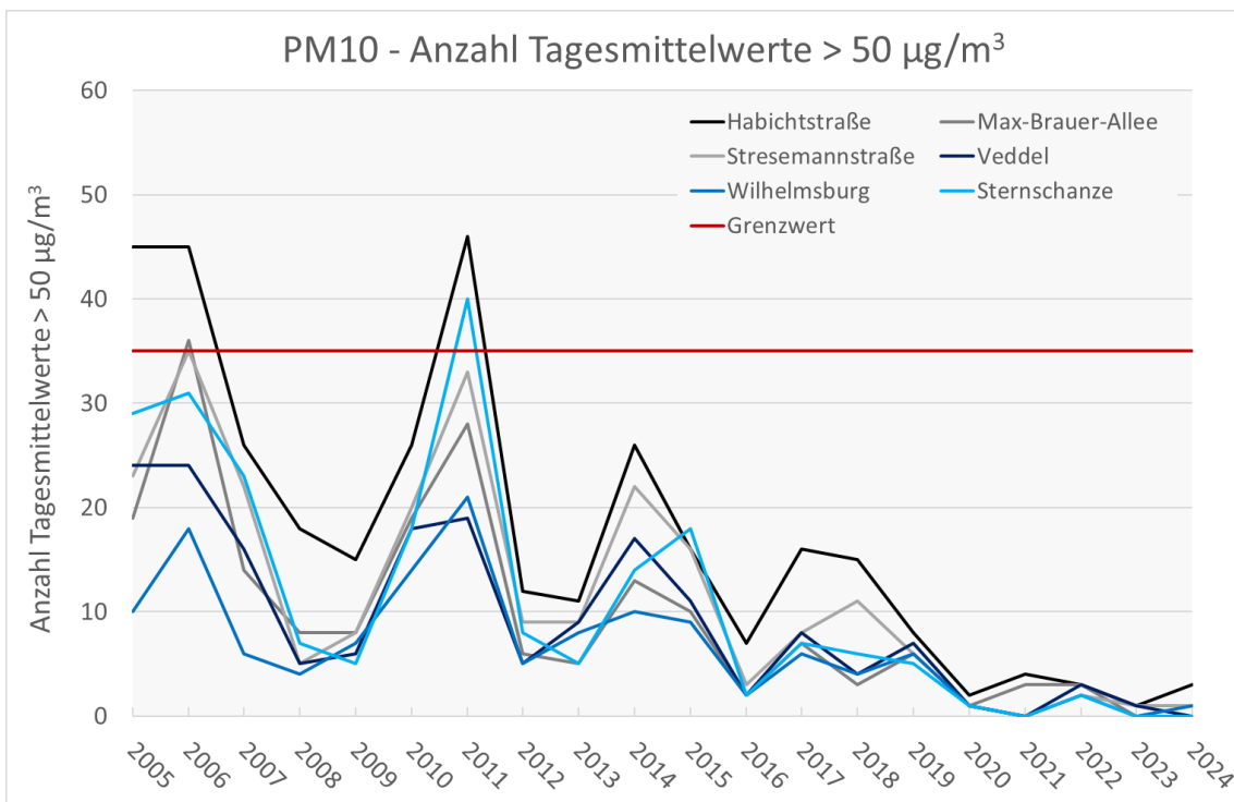
Abbildung 13: Anzahl an Tagesmittelwerten mit PM10-Konzentrationen > 50 \mu\text{g}/\text{m}^3 der Jahre 2005 bis 2024 an Messstationen zum Vollzug der 39. BImSchV in Hamburg.
