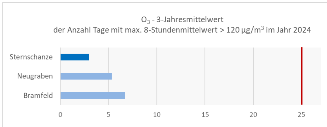
Abbildung 17: 3-Jahresmittelwerte der Jahre 2022 bis 2024 der Anzahl an Tagen mit 8-Stundenmittelwerten mit bodennahen Ozonkonzentrationen > 120 \mu\text{g}/\text{m}^3 an den Messstationen zum Vollzug der 39. BImSchV in Hamburg.
