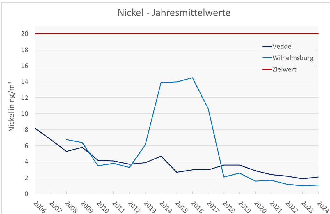
Abbildung 32: Jahresmittelwerte der Konzentration an Nickel in PM10 in ng/m 3 der Jahre 2006 bis 2024 an Messstationen zum Vollzug der 39. BImSchV in Hamburg.
