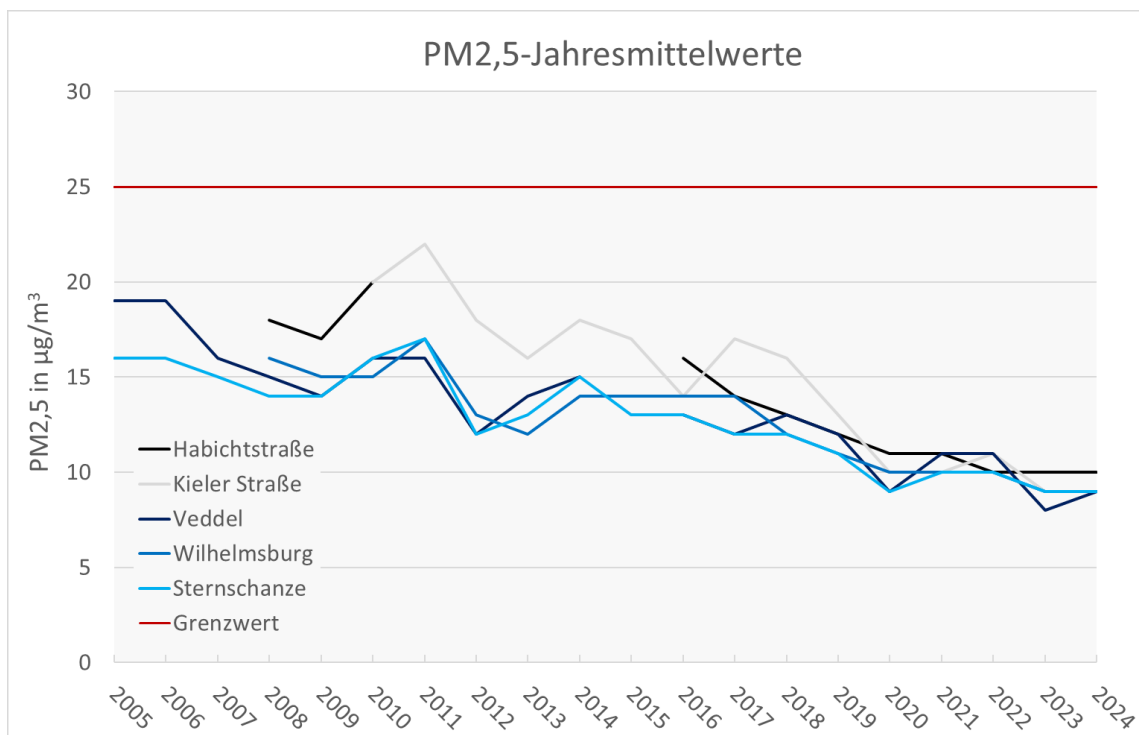
Abbildung 15: Jahresmittelwerte der PM 2,5 -Konzentration in µg/m 3 der Jahre 2005 bis 2024 an Messstationen zum Vollzug der 39. BImSchV in Hamburg.
