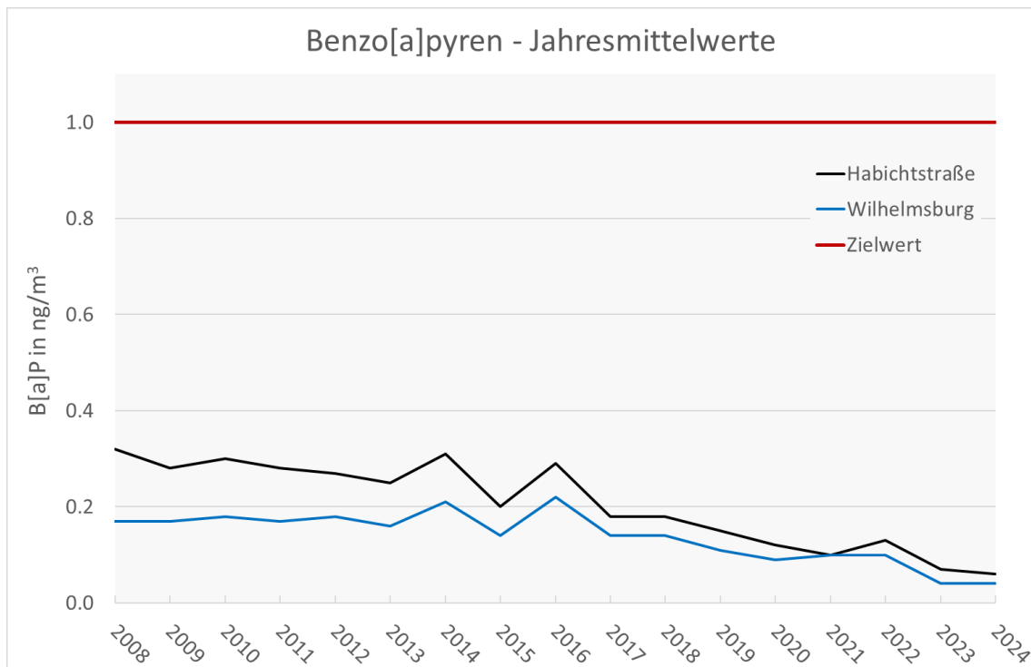
Abbildung 33: Jahresmittelwerte der Konzentration an Benzo(a)pyren in PM10 in ng/m 3 der Jahre 2008 bis 2024 an Messstationen zum Vollzug der 39. BImSchV in Hamburg.
