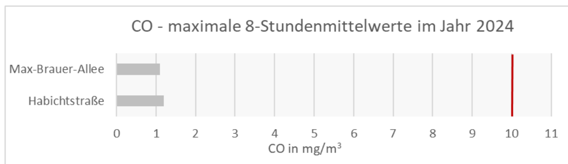
Abbildung 25: Maximale 8-Stundenmittelwerte der Kohlenstoffmonoxid-Konzentrationen in \text{mg/m}^3 an den Messstationen zum Vollzug der 39. BImSchV in Hamburg im Jahr 2024.
