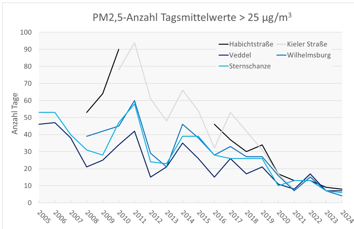
Abbildung 16: Anzahl an Tagsmittelwerten mit PM2,5 Konzentrationen > 25 µg/m 3 der Jahre 2005 bis 2024 an Messstationen zum Vollzug der 39. BImSchV in Hamburg.
