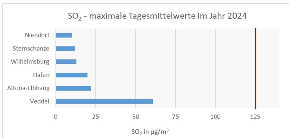
Abbildung 21: Maximale Tagesmittelwerte der Schwefeldioxidkonzentrationen in µg/m 3 an den Messstationen zum Vollzug der 39. BImSchV in Hamburg im Jahr 2024.
