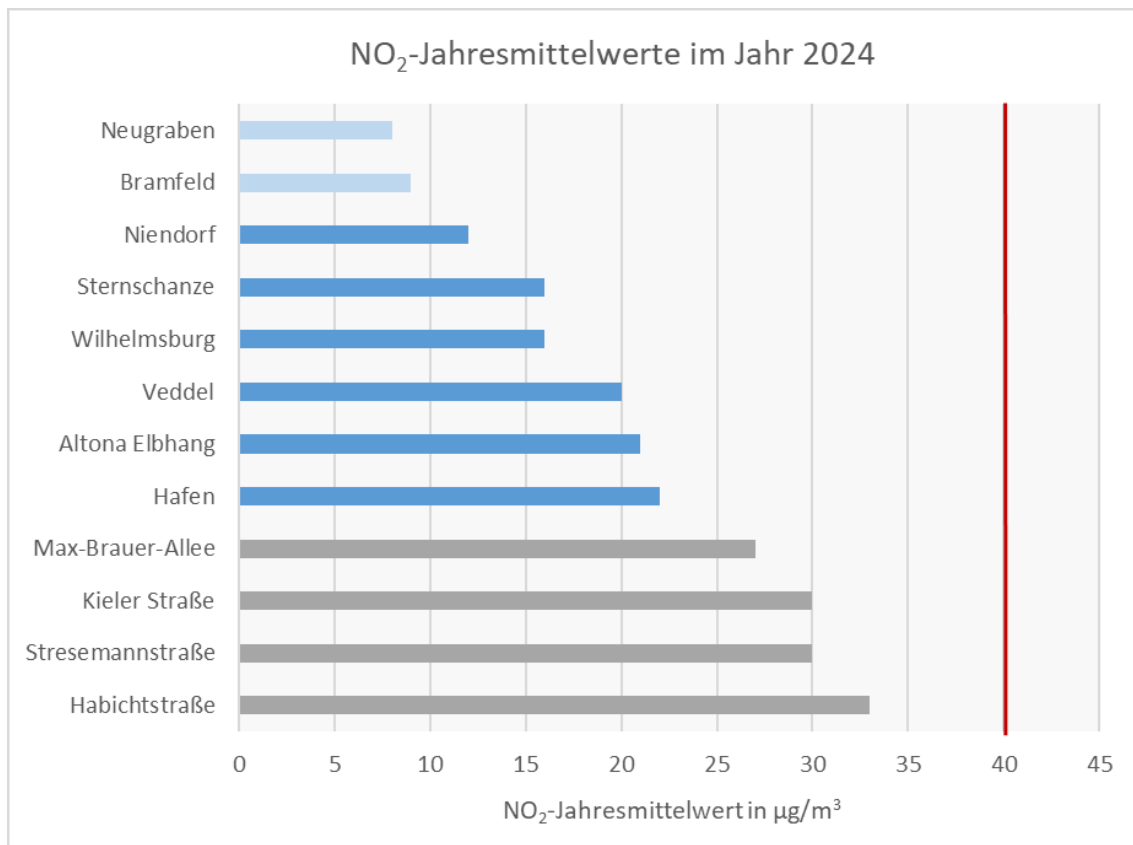
Abbildung 6: Jahresmittelwerte der Stickstoffdioxidkonzentration in \mu\text{g}/\text{m}^3 an den Messstationen zum Vollzug der 39. BImSchV in Hamburg im Jahr 2024.
