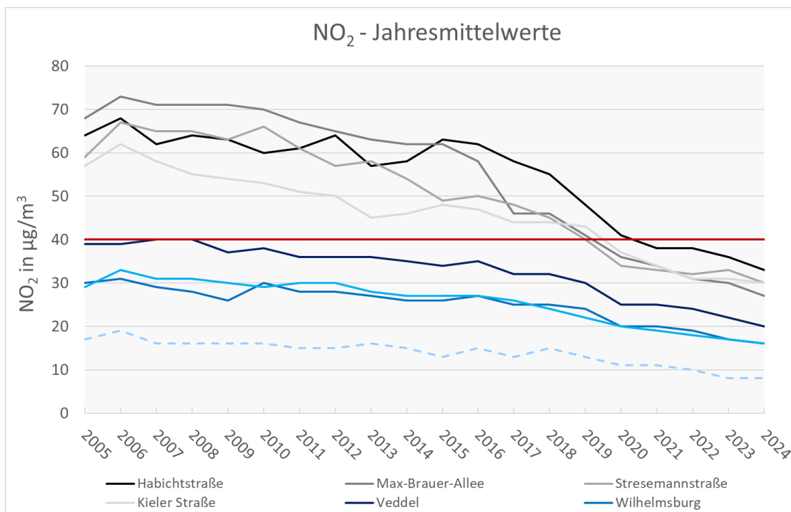
Abbildung 8: Jahresmittelwerte der Stickstoffdioxidkonzentration in \mu\text{g}/\text{m}^3 der Jahre 2005 bis 2024 an Messstationen zum Vollzug der 39. BImSchV in Hamburg, verkehrsnahen Messstationen in 1,5 m Messhöhe.
