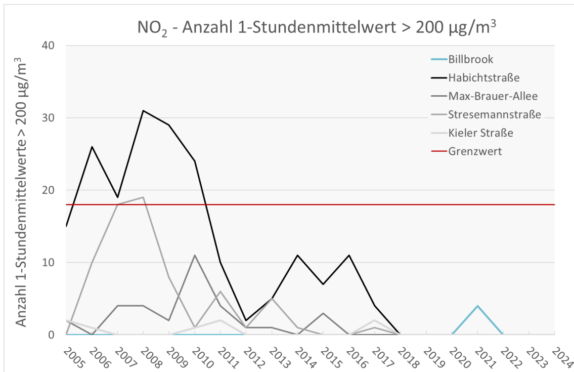
Abbildung 9: Anzahl an 1-Stundenmittelwerten mit NO 2 -Konzentrationen > 200 µg/m 3 der Jahre 2005 bis 2024 an verkehrsnahen Messstationen zum Vollzug der 39. BImSchV in Hamburg (1,5 m Messhöhe) und an der Station Billbrook.
