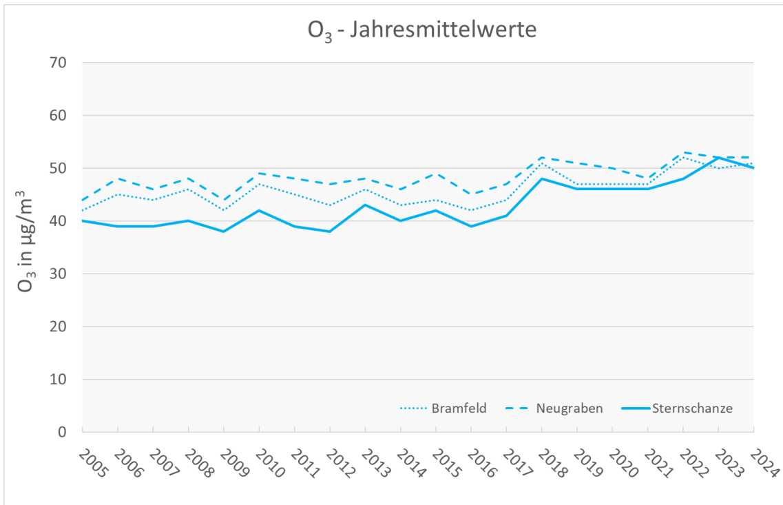
Abbildung 18: Jahresmittelwerte der Ozon-Konzentration in \mu\text{g}/\text{m}^3 der Jahre 2005 bis 2024 an den Messstationen zum Vollzug der 39. BImSchV in Hamburg.
