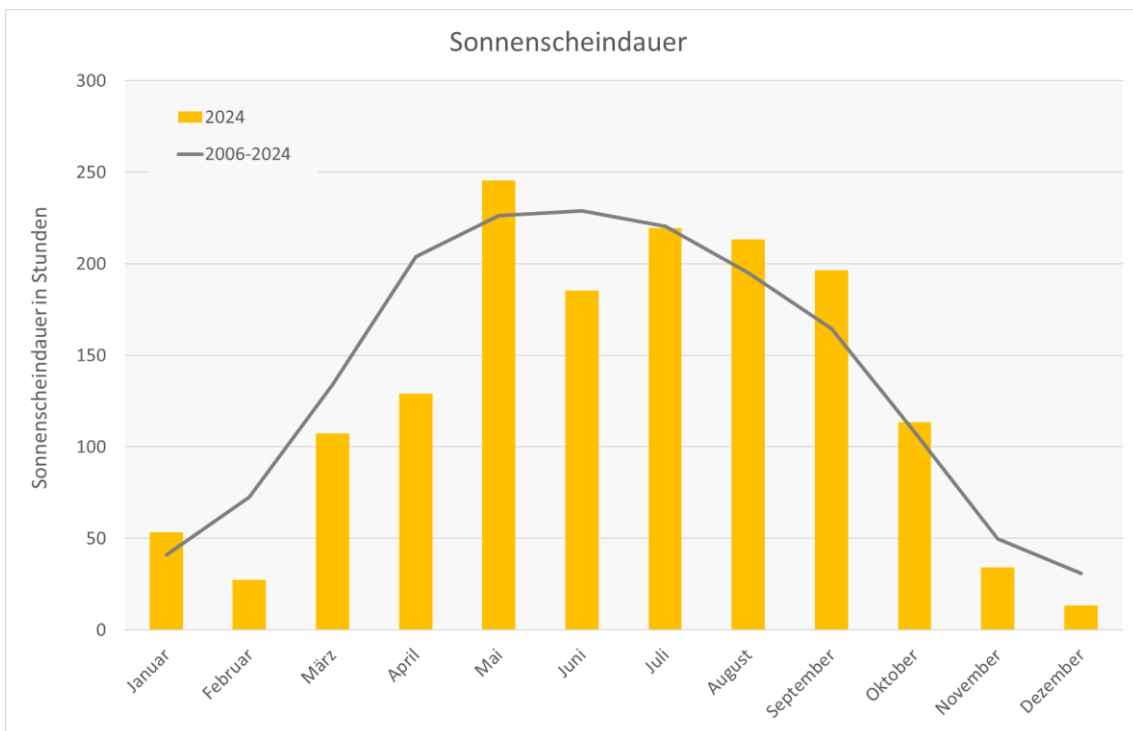
Abbildung 4: Monatssummen der Sonnenscheindauer in h am Wettermast Hamburg im Jahr 2024 (gelbe Balken) und Mittelwert der Jahre 2006-2024 (graue Linie). Datenquelle: Universität Hamburg.
