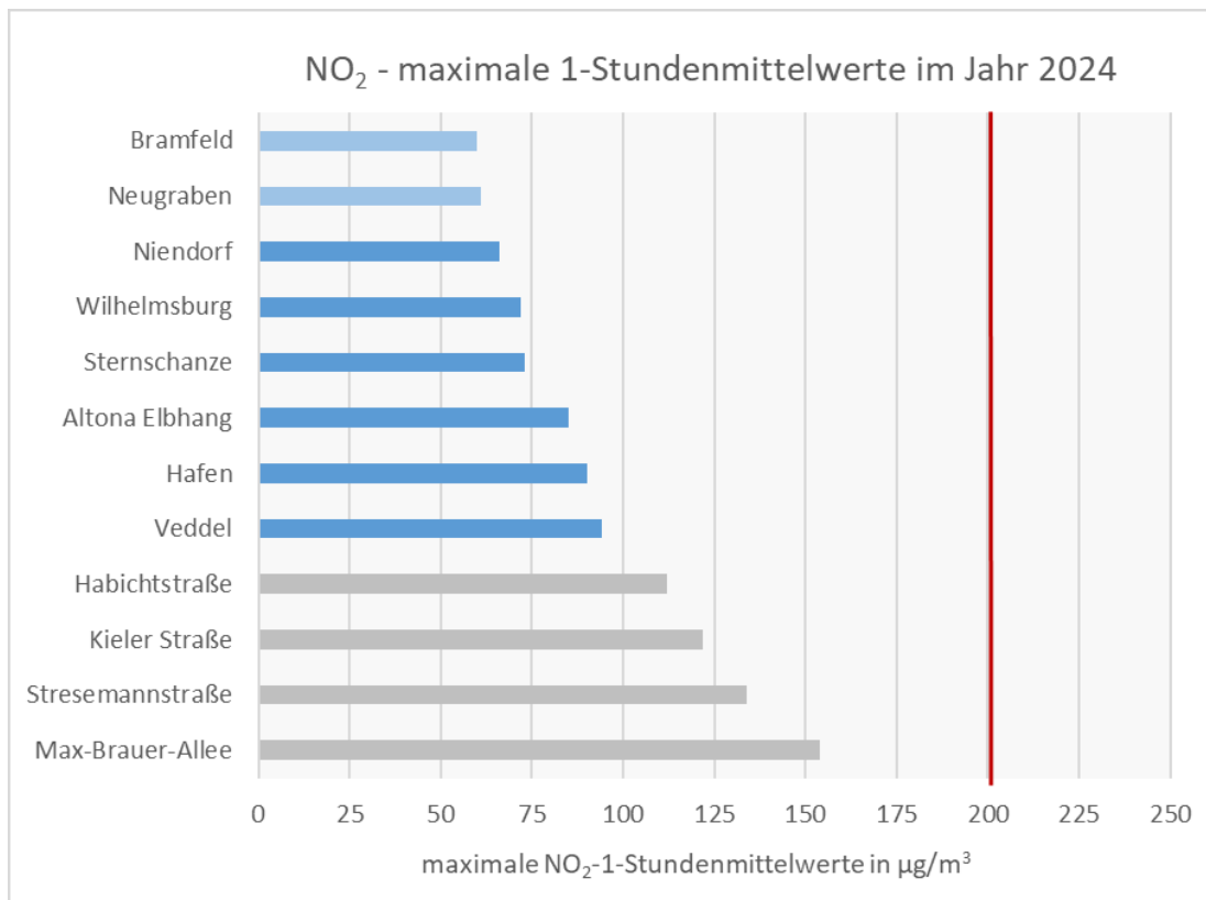
Abbildung 7: Maximale 1-Stundenmittelwerte der Stickstoffdioxidkonzentration in µg/m 3 an den Messstationen zum Vollzug der 39. BImSchV in Hamburg im Jahr 2024 im Vergleich zum Grenzwert (rote Linie).
