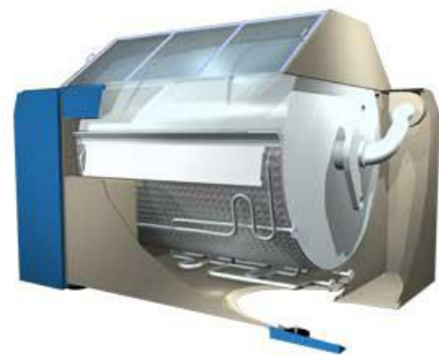
Die Mangel HPM 20 – G 3000 (Abb. aus dem Internetauftritt der Firma Kannegießer ( www.kannegiesser.de ))
