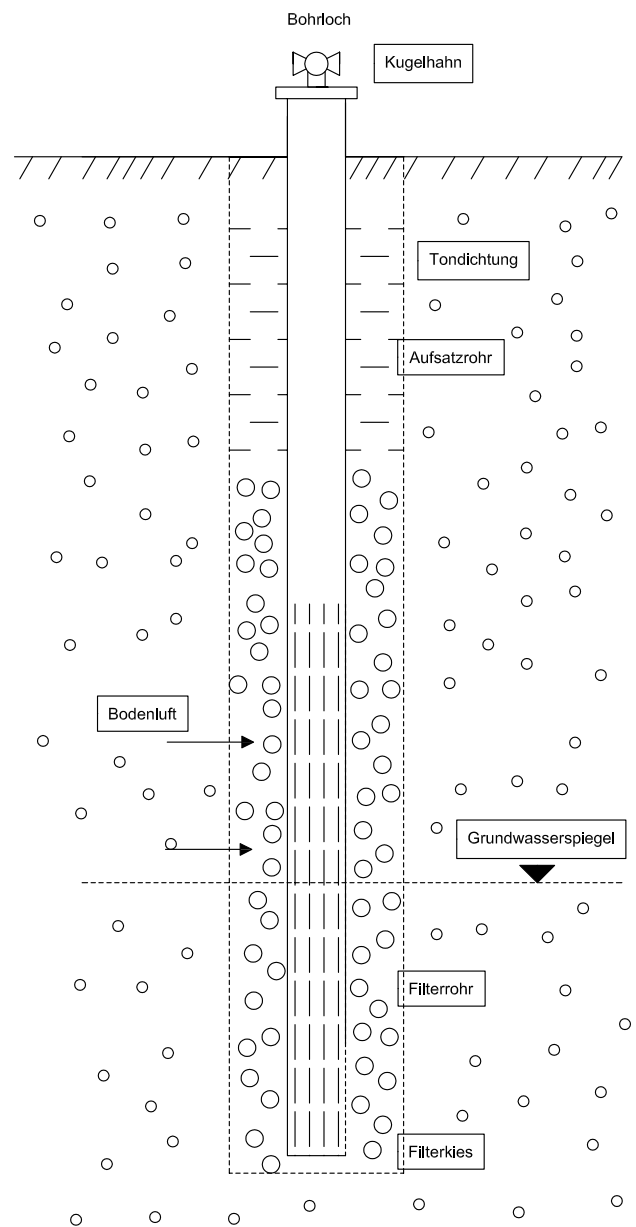
Abbildung 3: Prinzipskizze einer stationären kombinierten Grundwasser- und Bodenluft-/Deponiegasmessstelle
