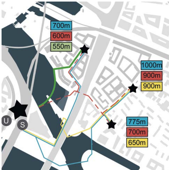
Planungsvarianten zur Querung der Billhorner Brückenstraße
