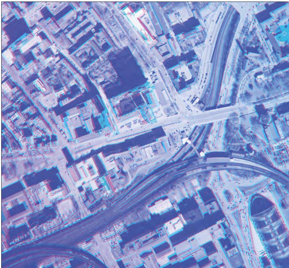
Das Anaglyphenbild von 2006 zeigt die Umgebung beim S-Bahnhof Berliner Tor. Beim Betrachten mit der Rot-Grün-Brille sieht man deutlich den Taleinschnitt, die Brückenbauten und die unterschiedlichen Gebäudehöhen
