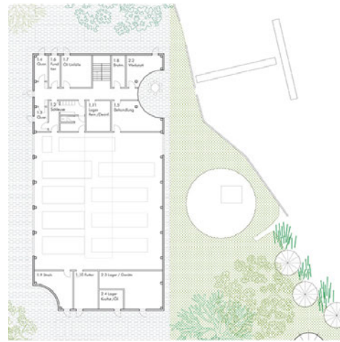
Grundriss EG
