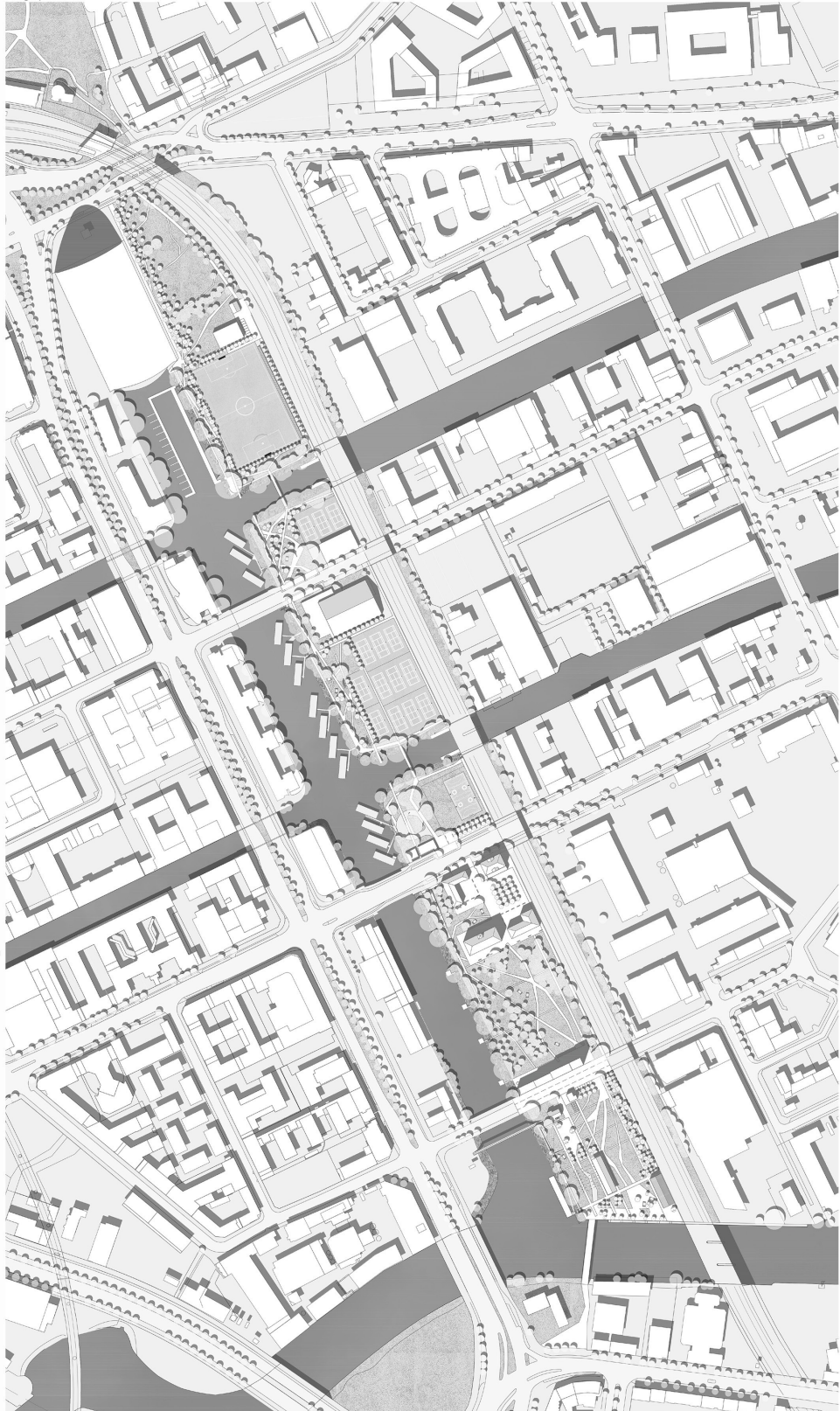
Lageplan M 1: 2000
